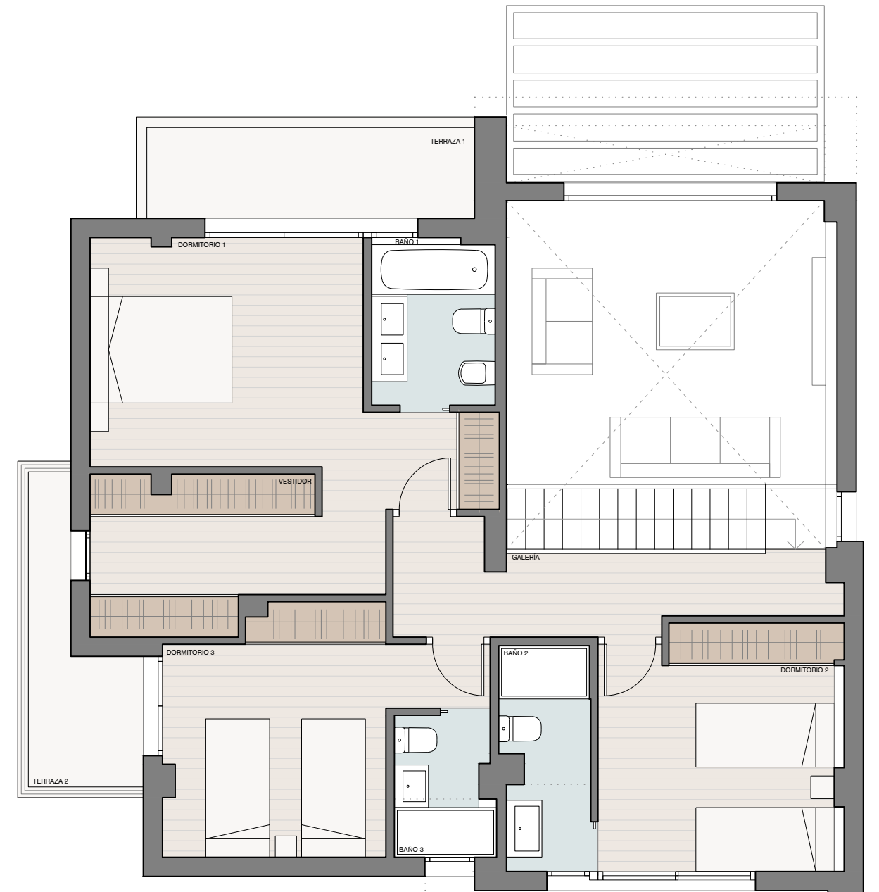
PLANTA SUPERIOR
